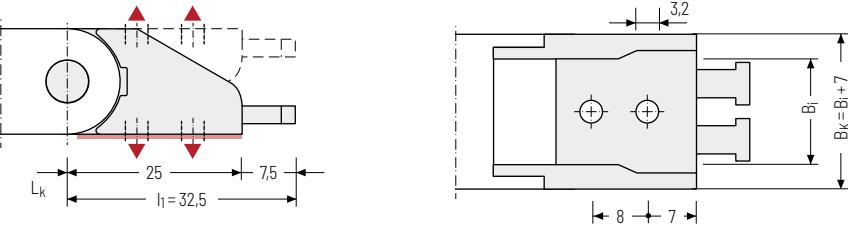
▲ Montagemöglichkeiten
